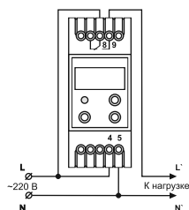
Схема подключения
