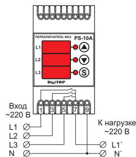
Схема подключения
