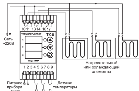
Схема подключения
