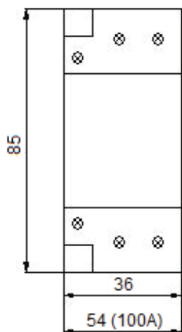
МК-N 2P (32, 100A)
