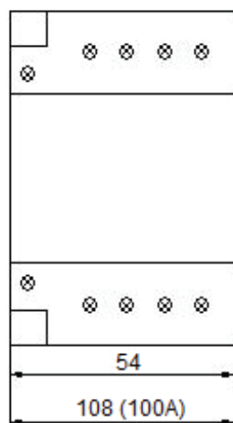
МК-N 4P (32, 40, 63, 100A)
