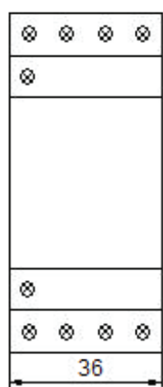
МК-N 4P (16, 20, 25A)
