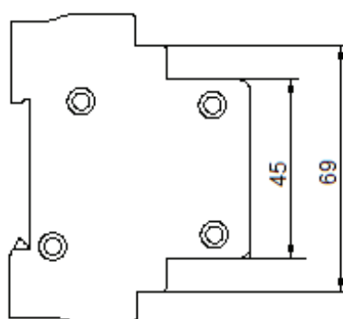
МК-N 4P (32, 40, 63, 100A)
