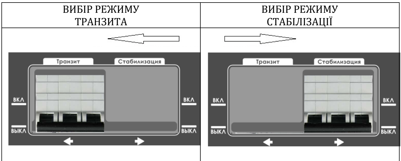
Рисунок 7. Порядок переключення між режимами роботи стабілізатору
