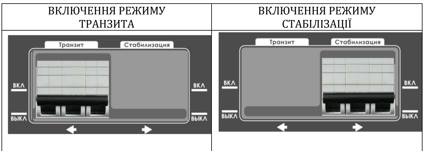
Рисунок 8. Положення тумблеру автоматичного вимикача при виборі режиму роботи
