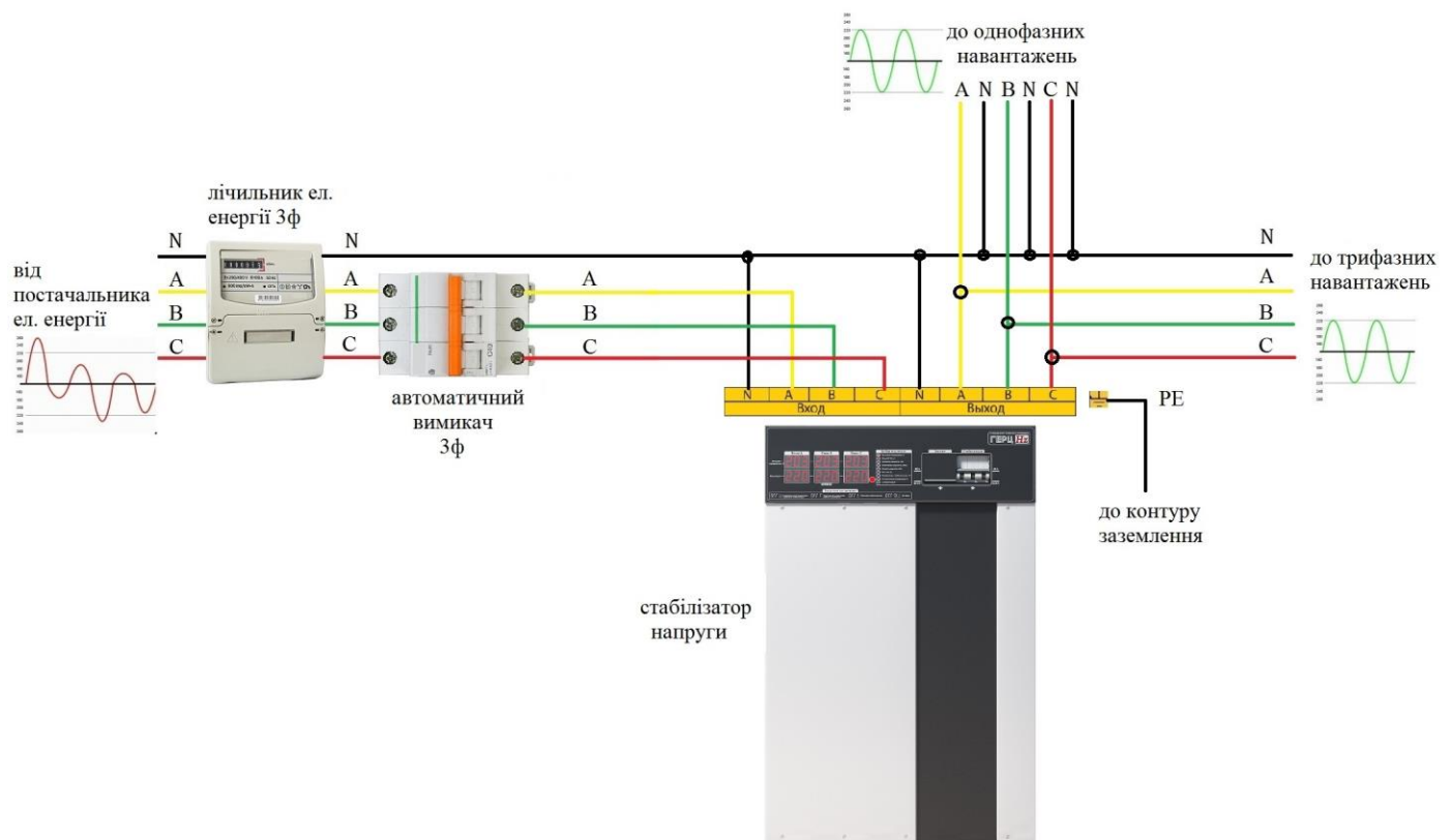
Рисунок 5. Схема підключення стабілізатора до трифазної мережі
