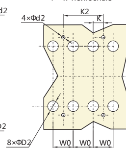
4 - х полюсные
