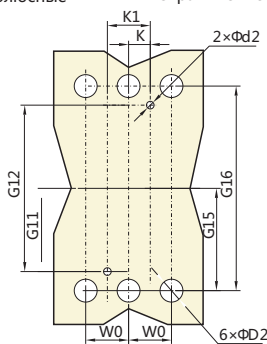
3 - х полюсные
