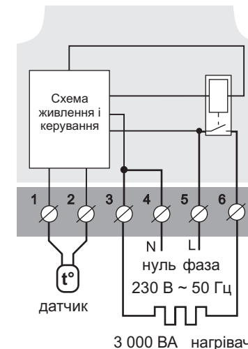
Схема 1. Схема підключення та спрощена внутрішня схема
